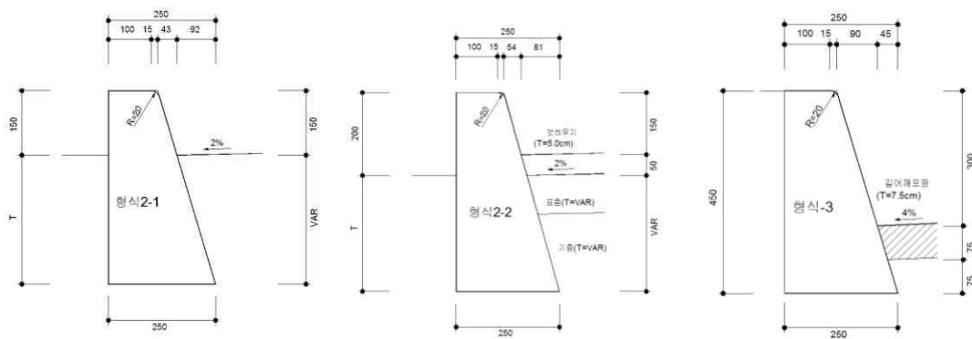
<콘크리트 다이크 Type 2-1, 2-2>
