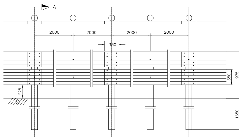
<1단 가드레일>
