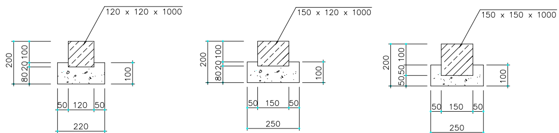
<경계블록>
