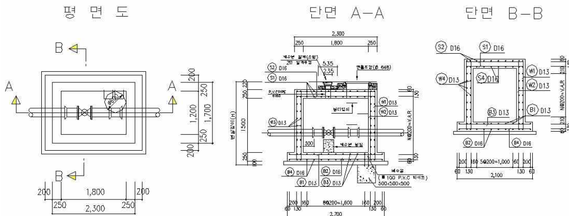
<제수변실(1.8m×1.2m)>
