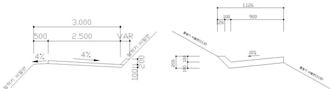
<소단측구 형식 1>
