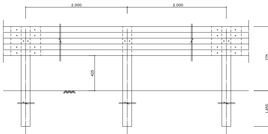
<1단 가드레일>
