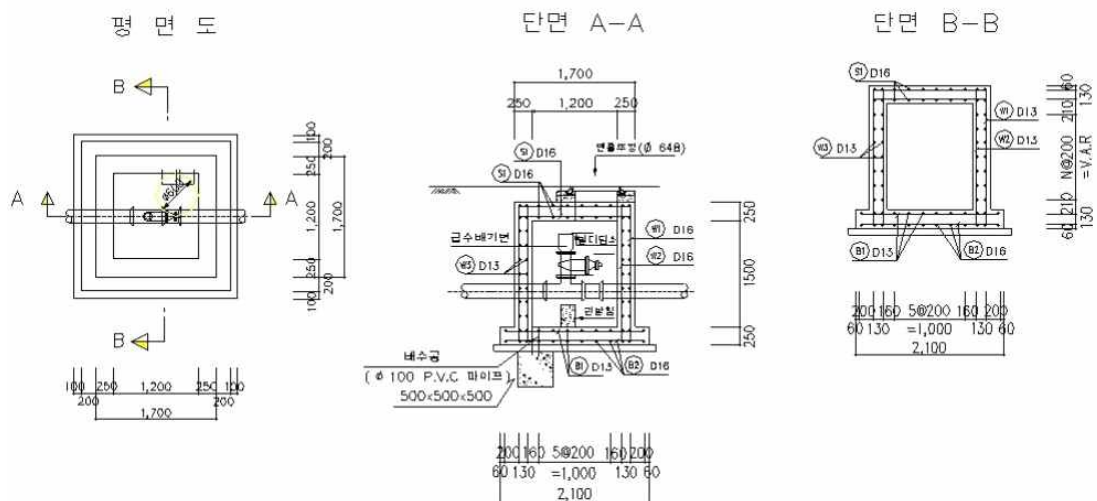
<공기변실(1.2m×1.2m)>
