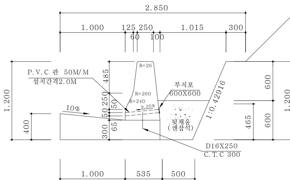
<L형측구 형식 2-고속국도>
