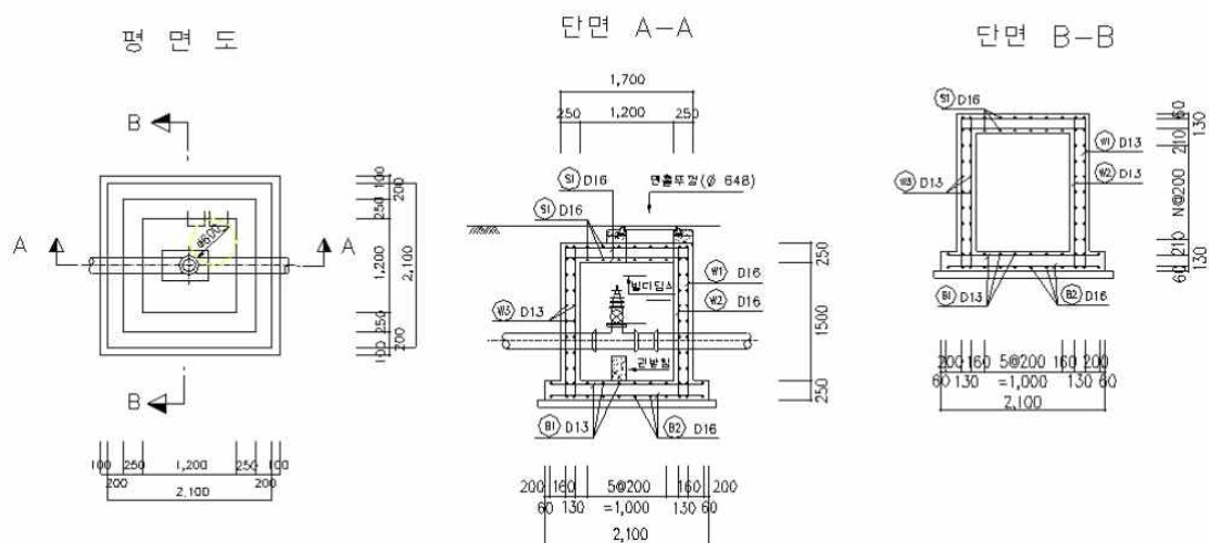
<이토변실(1.2m×1.2m)>
