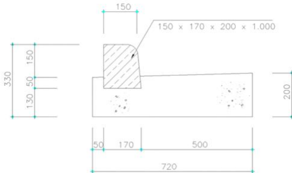
<보차도 경계블록(콘크리트)>
