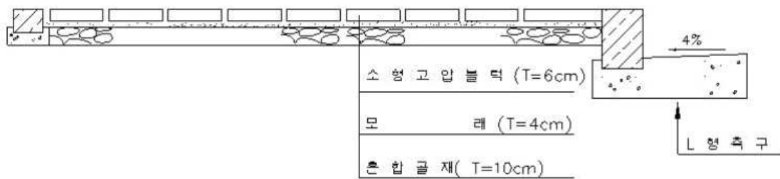
<소형고압블록>
