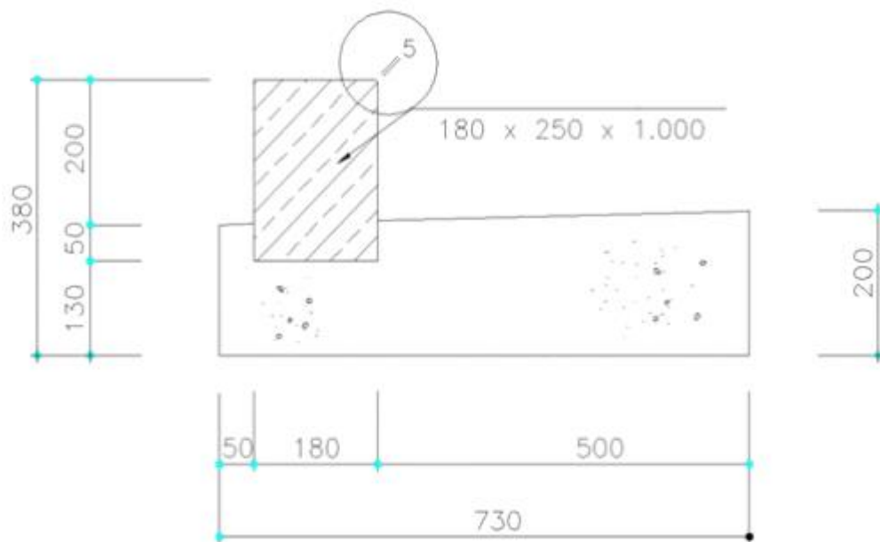
<보차도 경계석(화강석)>
