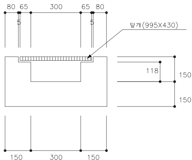
<U형측구 형식 1>
