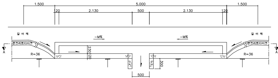
<다이크 집수거 L형>
