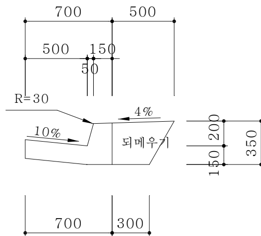
<L형측구 형식 4-고속국도>
