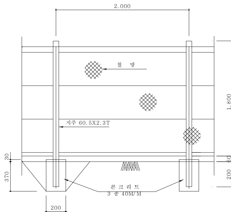
<가드휀스-토공용>
