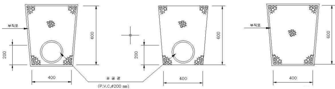
<맨암거 형식-1><맨암거 형식-2>
