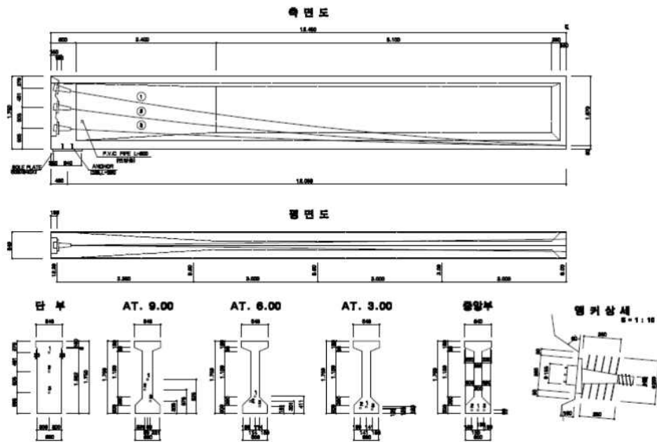
<PSC BEAM(L=25m) 표준도>
