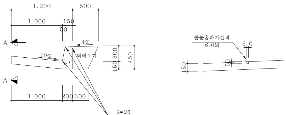
<L형측구 형식 1-고속국도>
