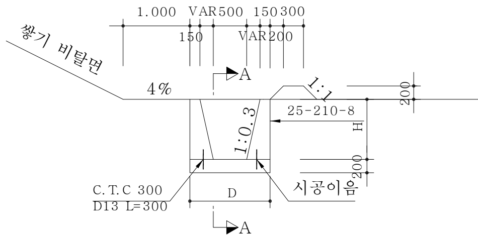
<V형측구 형식 1,2,3>
