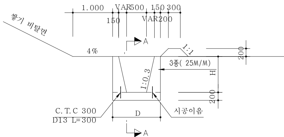
<V형측구 형식 1,2,3-고속국도>
